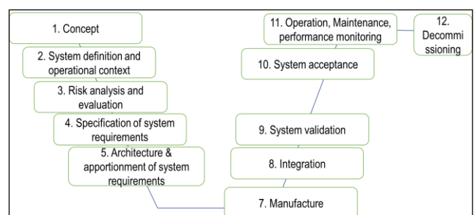
図 1 EN 50126 のライフサイクルモデル
