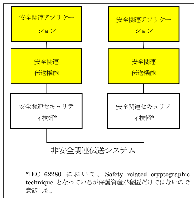
図 5 IEC 62280 における伝送参照モデル (黄色の部分安全関連系として管理することが要求されている)
