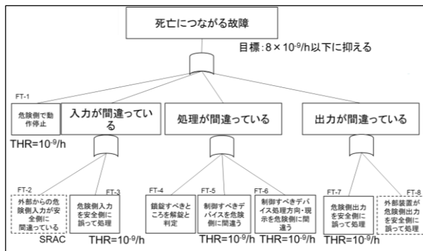
図 6 FTA 解析のイメージ
